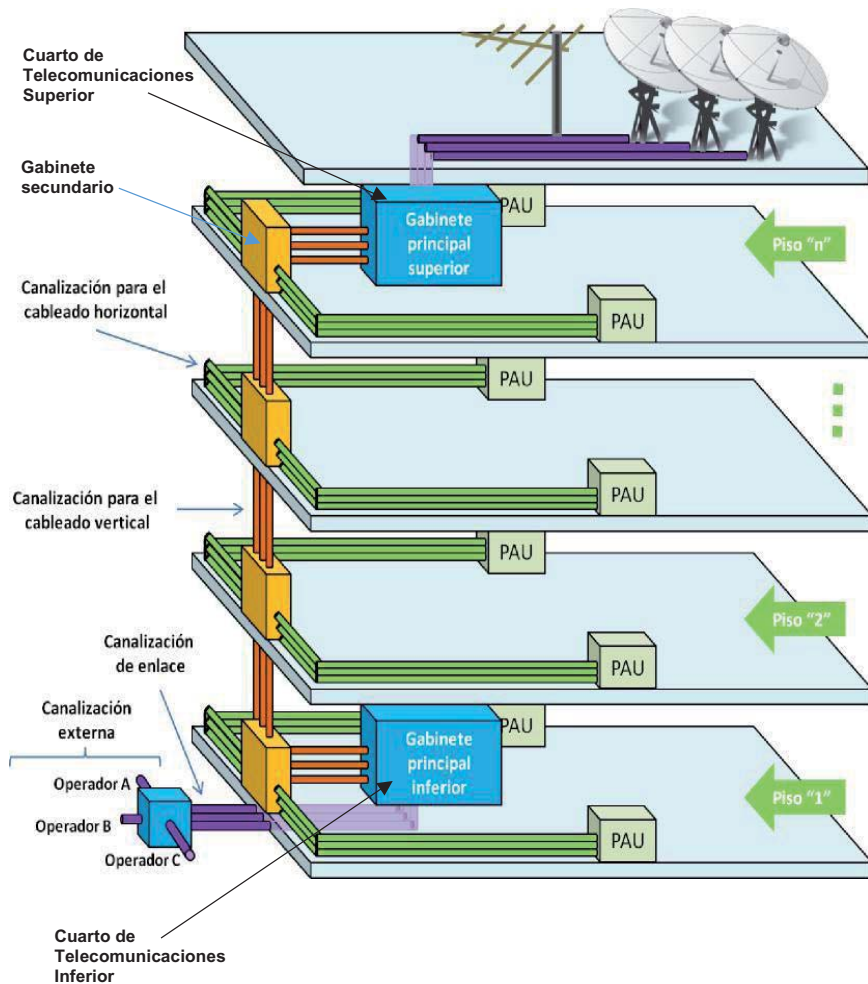
Gráfico 3 Esquema referencial de canalización de una edificación
